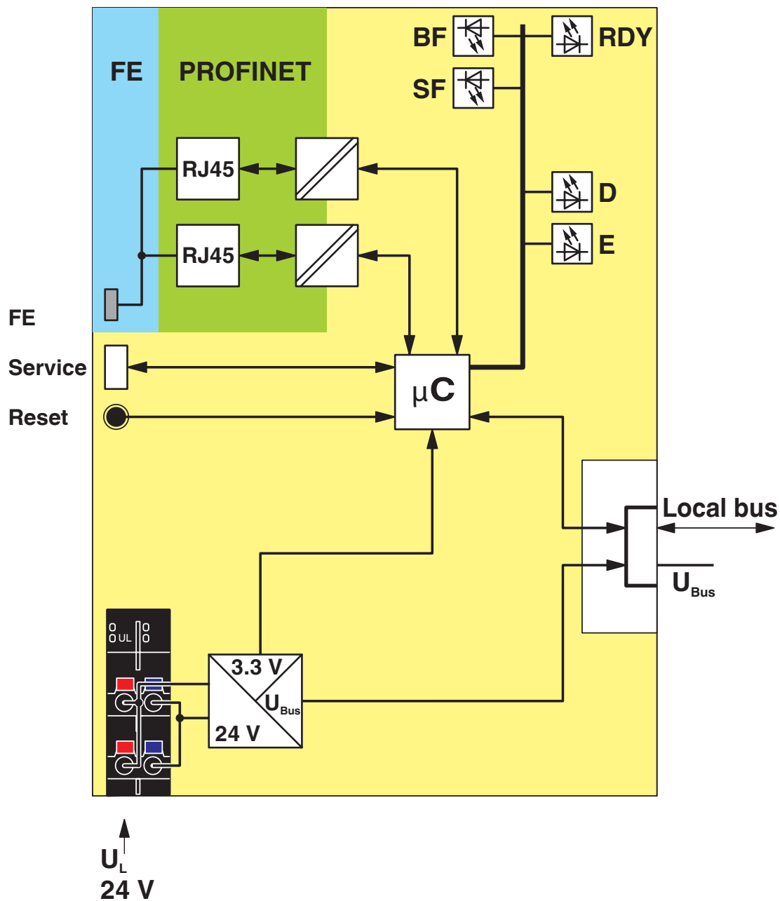
Blockschaltbild
