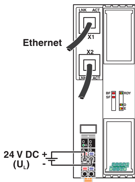
Anschlusszeichnung
