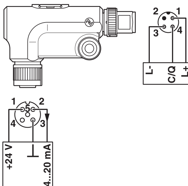
Anschlusszeichnung
