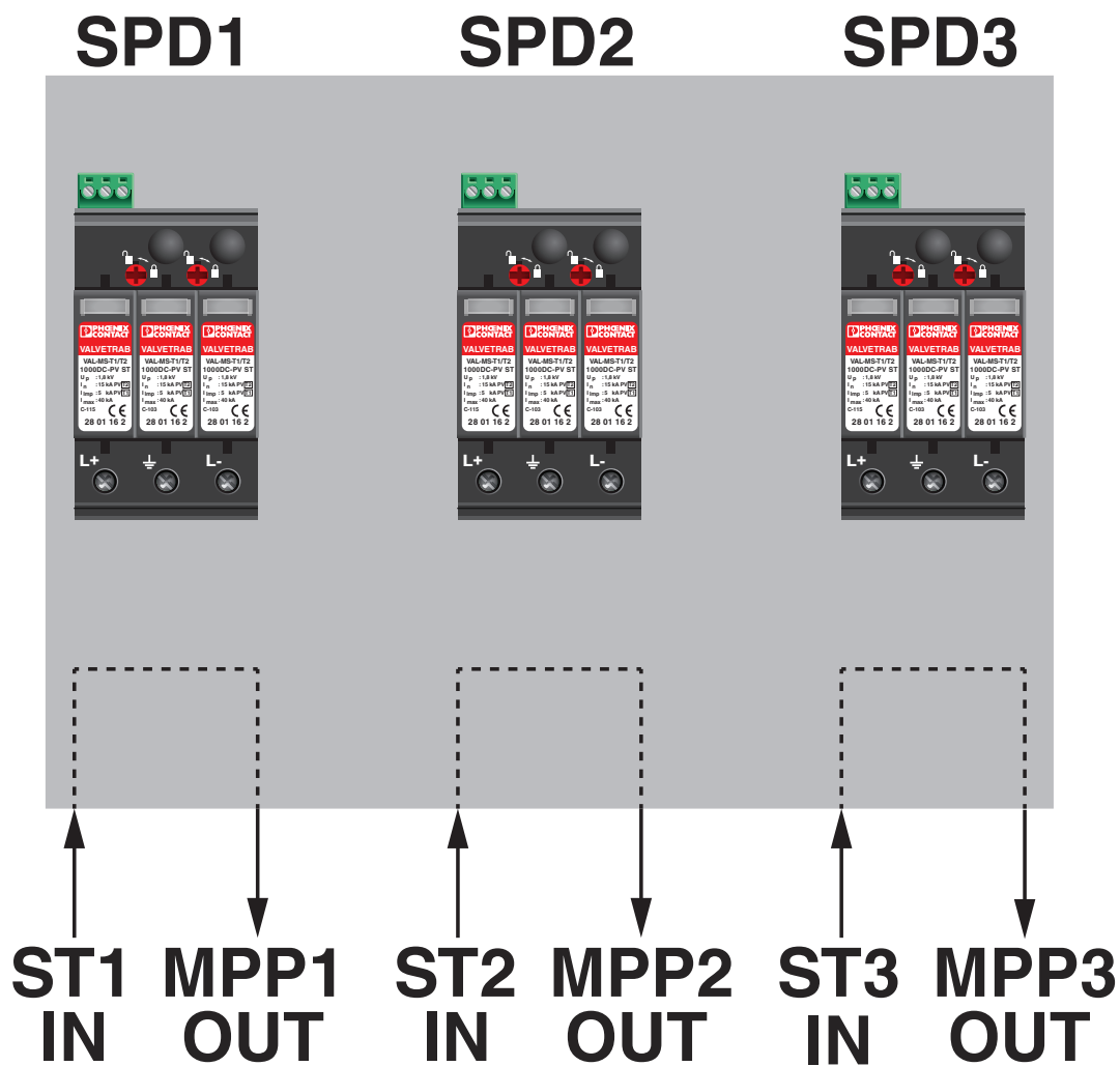
Schematische Applikationszeichnung
