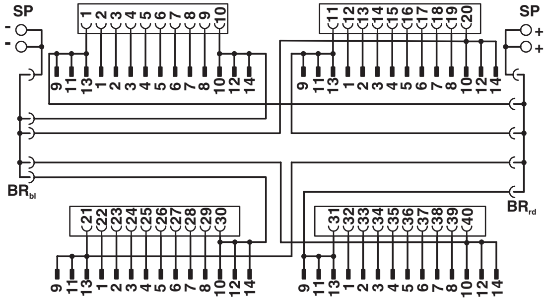
Schaltplan
