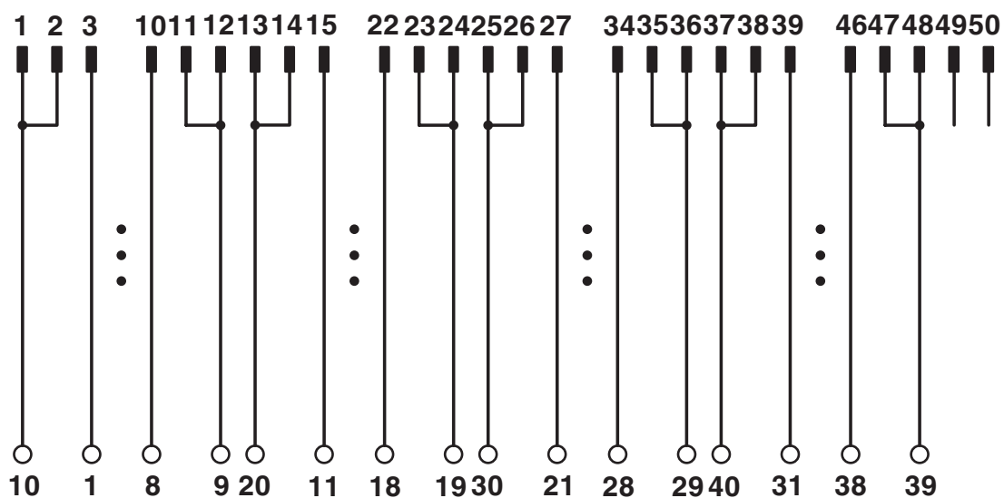
Anschlussbild VIP-2/.../FLK50/MODI-TSX/Q
