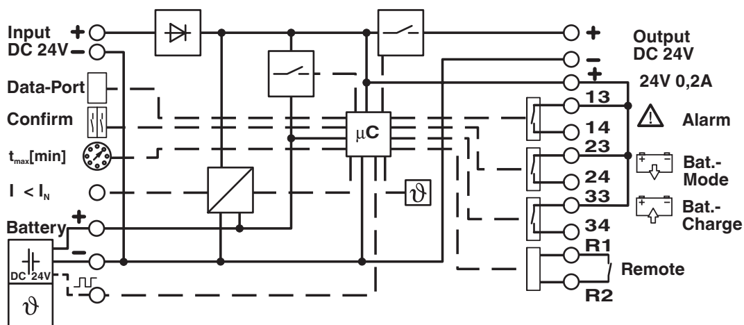
Blockschaltbild
