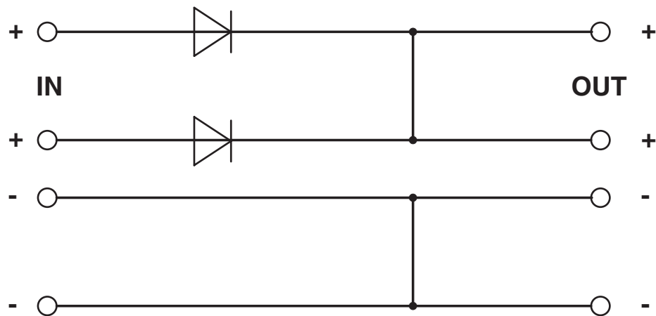
Blockschaltbild
