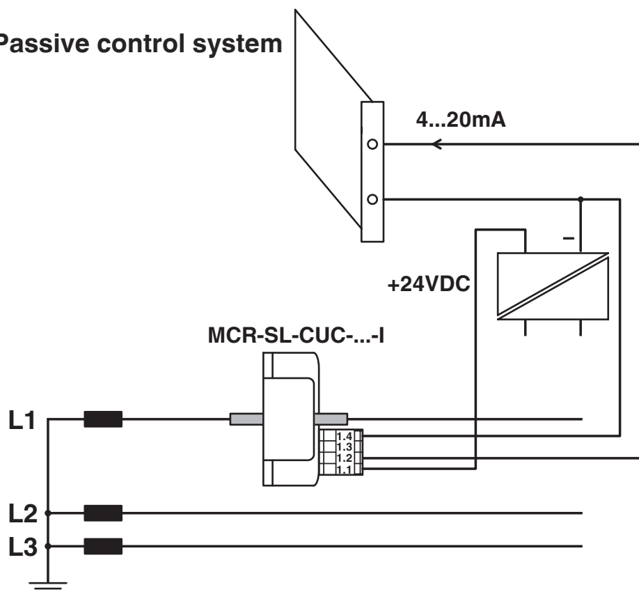
Applikationszeichnung
