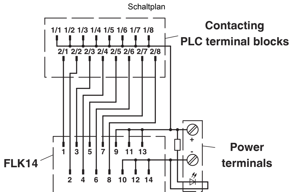
Anschlussbild PLC-V8L/FLK14/OUT/M
