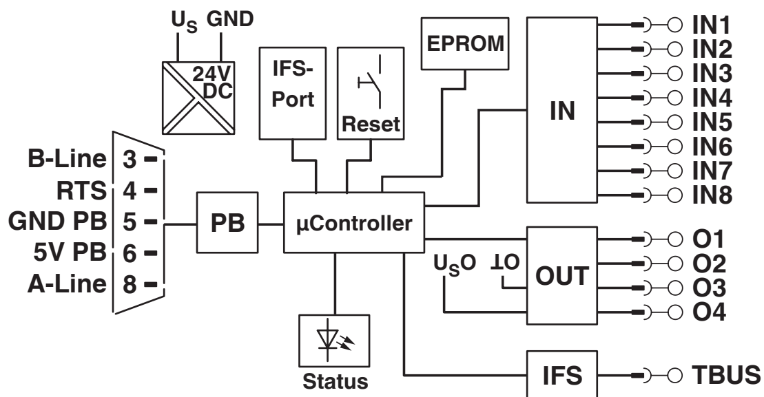
Blockschaltbild
