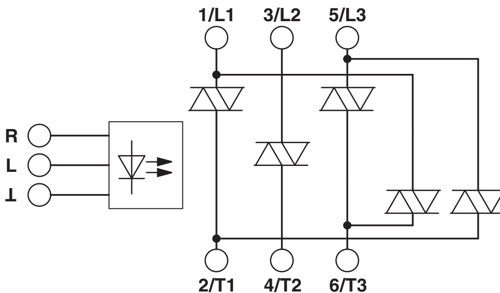
Blockschaltbild
