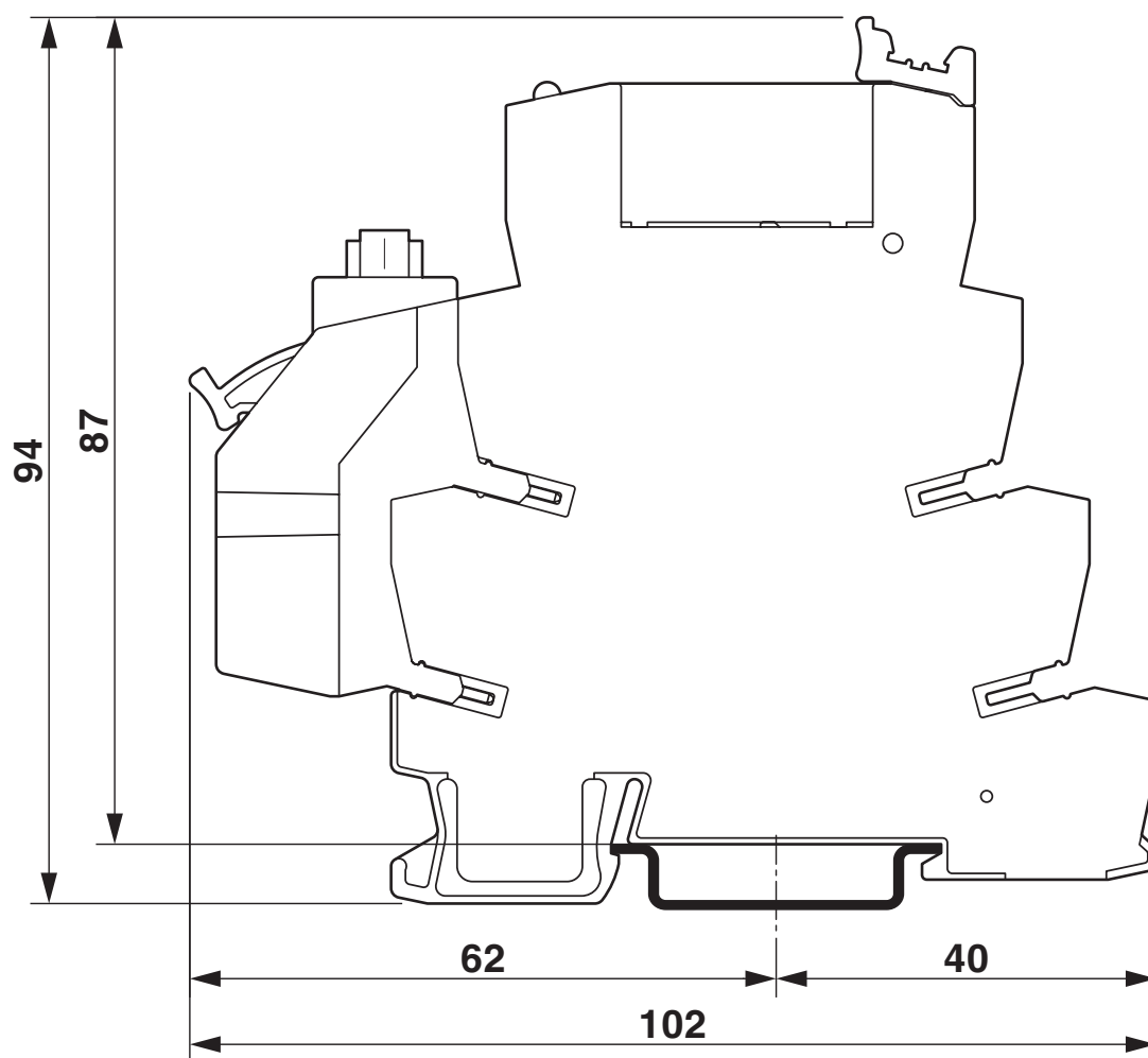
Maßzeichnung
