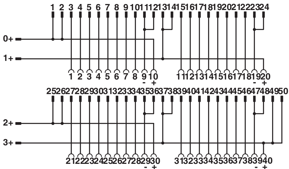
Anschlussbild FLKM 50-PA-MODI-TSX/Q
