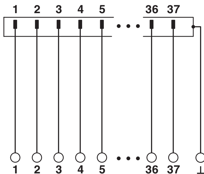
Schaltplan
