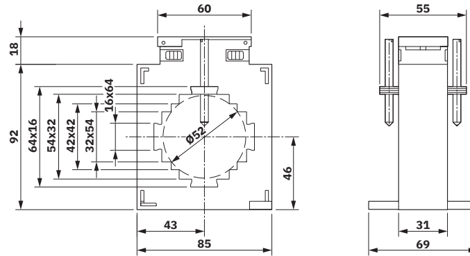
Maßzeichnung
