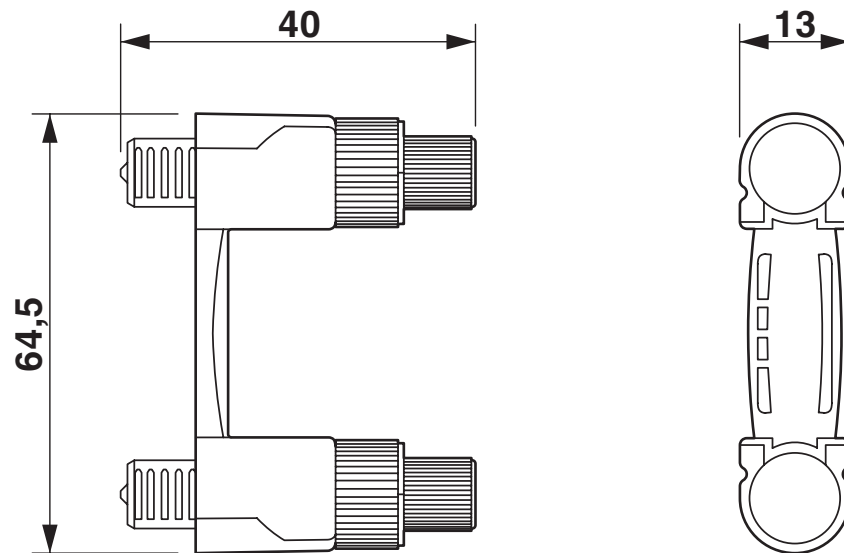
Maßzeichnung
