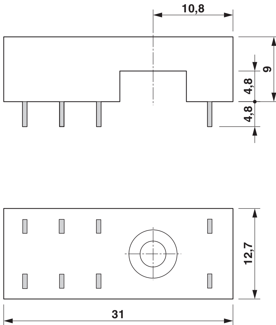
Maßzeichnung
