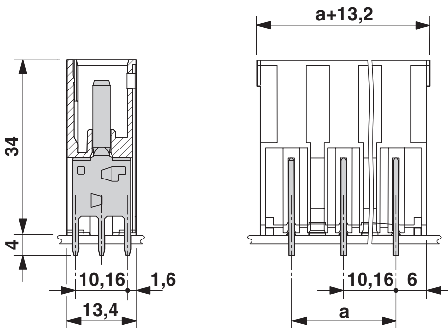
Maßzeichnung
