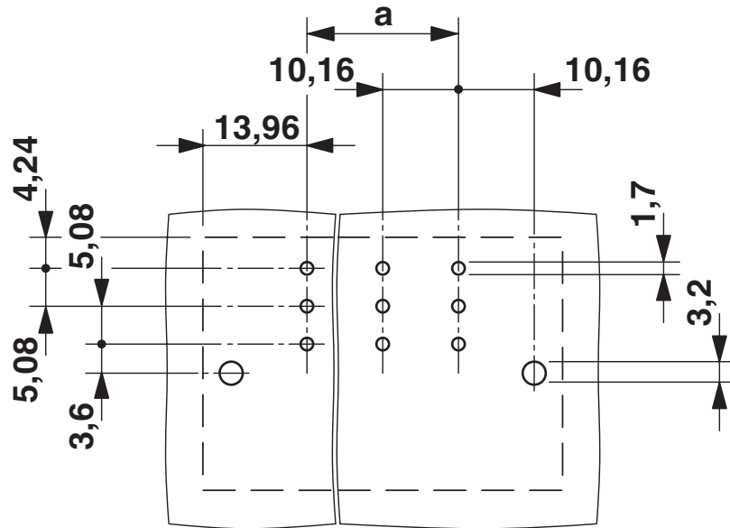
Bohrplan/Lötpadgeometrie
