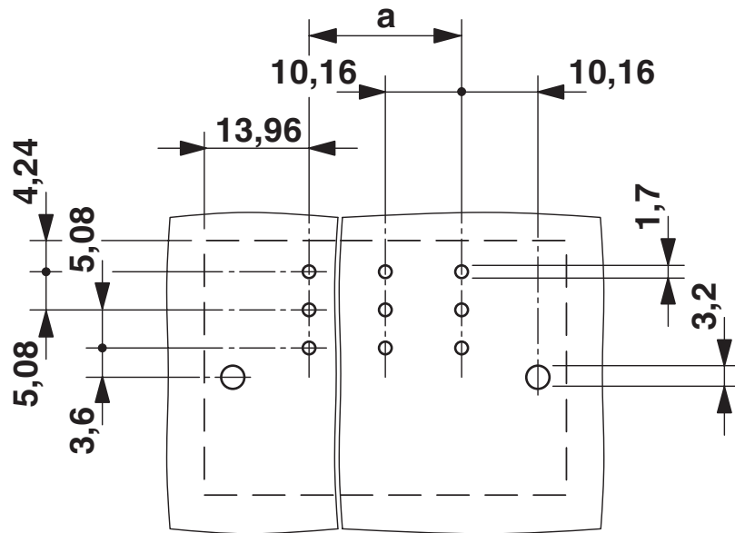
Bohrplan/Lötpadgeometrie
