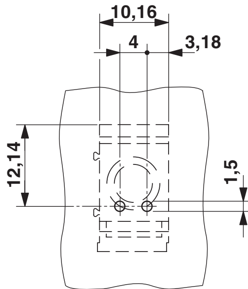
Bohrplan/Lötpadgeometrie
