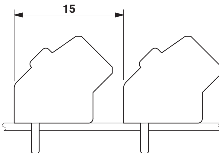
Maßzeichnung
