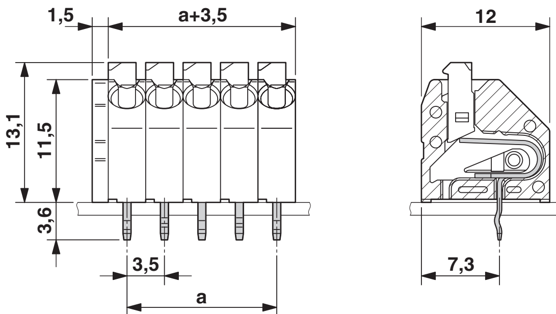
Maßzeichnung
