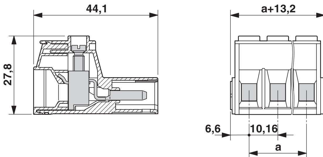
Maßzeichnung
