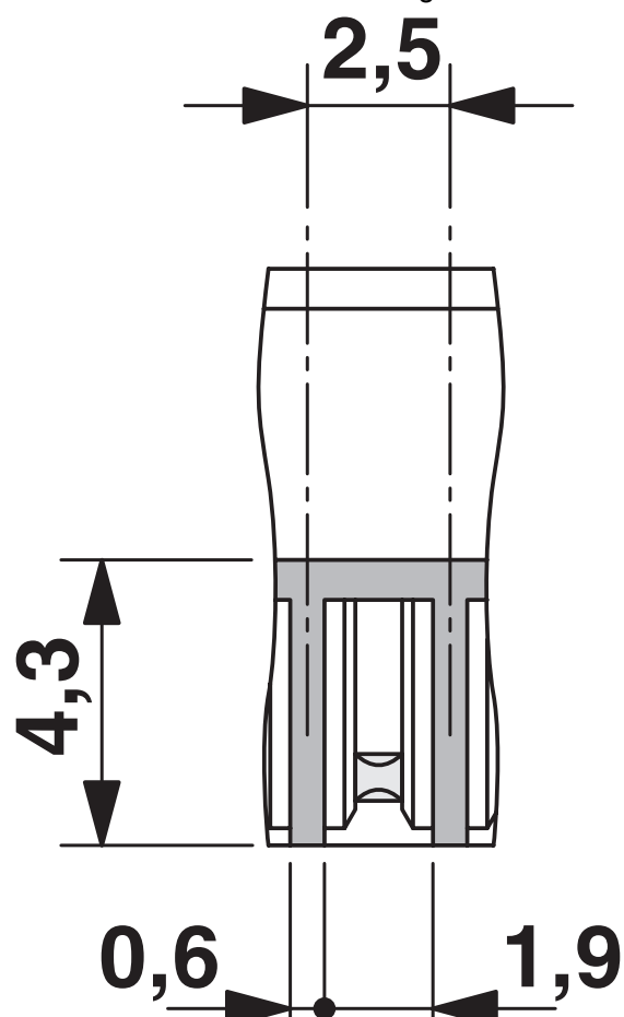
Maßzeichnung
