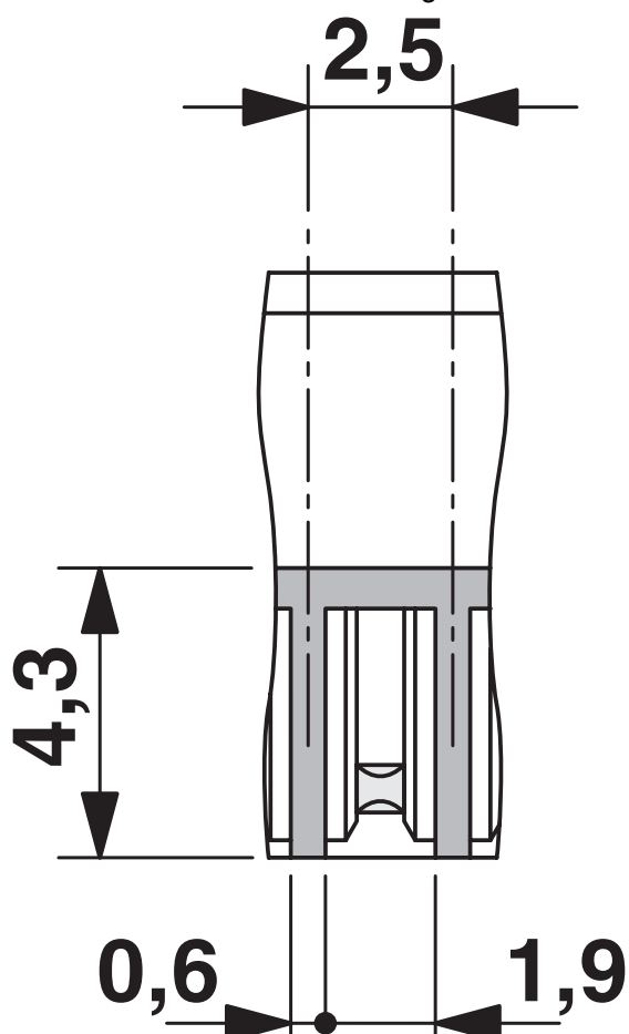
Maßzeichnung
