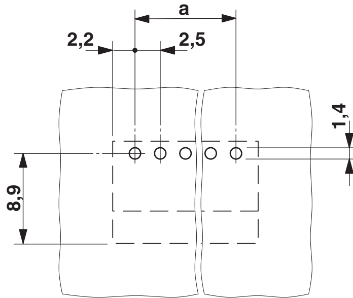
Bohrplan/Lötpadgeometrie
