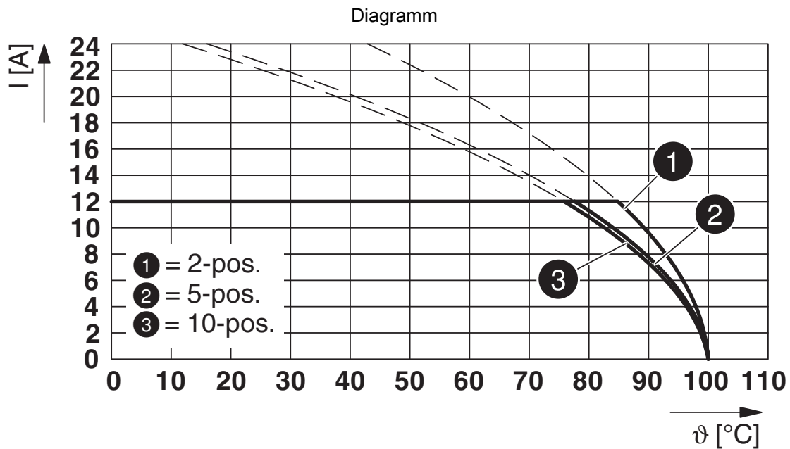
Typ: TFKC 2,5/...-ST-5,08 mit CCV 2,5/...-G-5,08 P...THR
