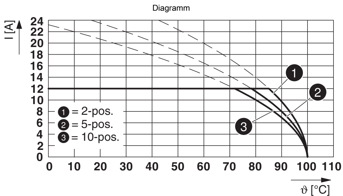
Typ: TFKC 2,5/...-ST-5,08 mit CCVA 2,5/...-G-5,08 P...THR
