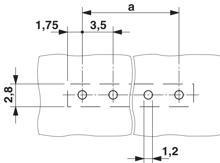
Bohrplan/Lötpadgeometrie
