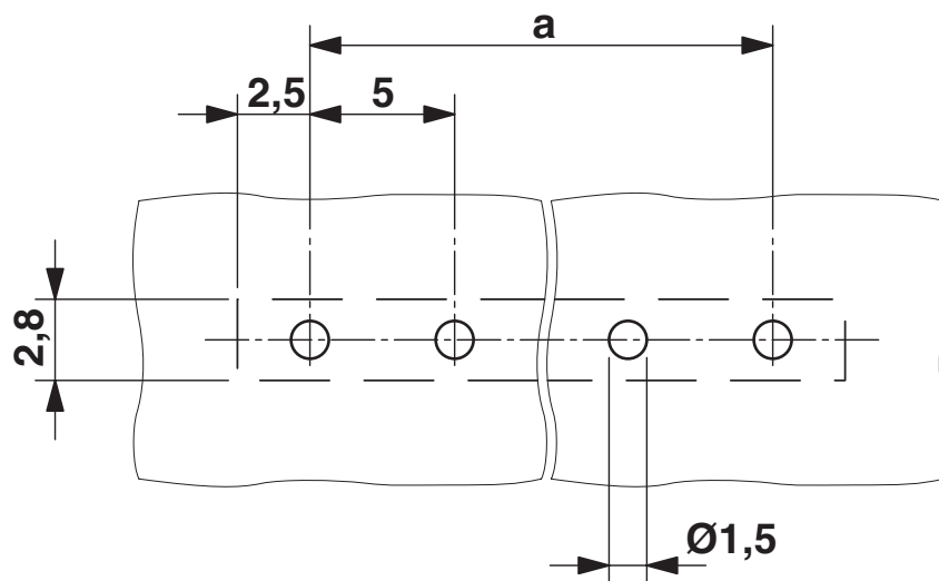
Bohrplan/Lötpadgeometrie
