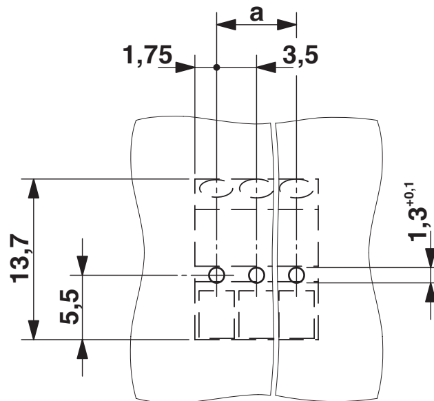
Bohrplan/Lötpadgeometrie
