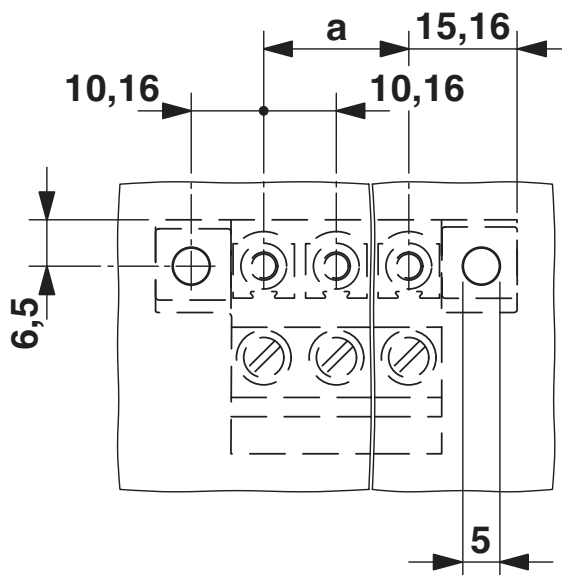
Bohrplan/Lötpadgeometrie
