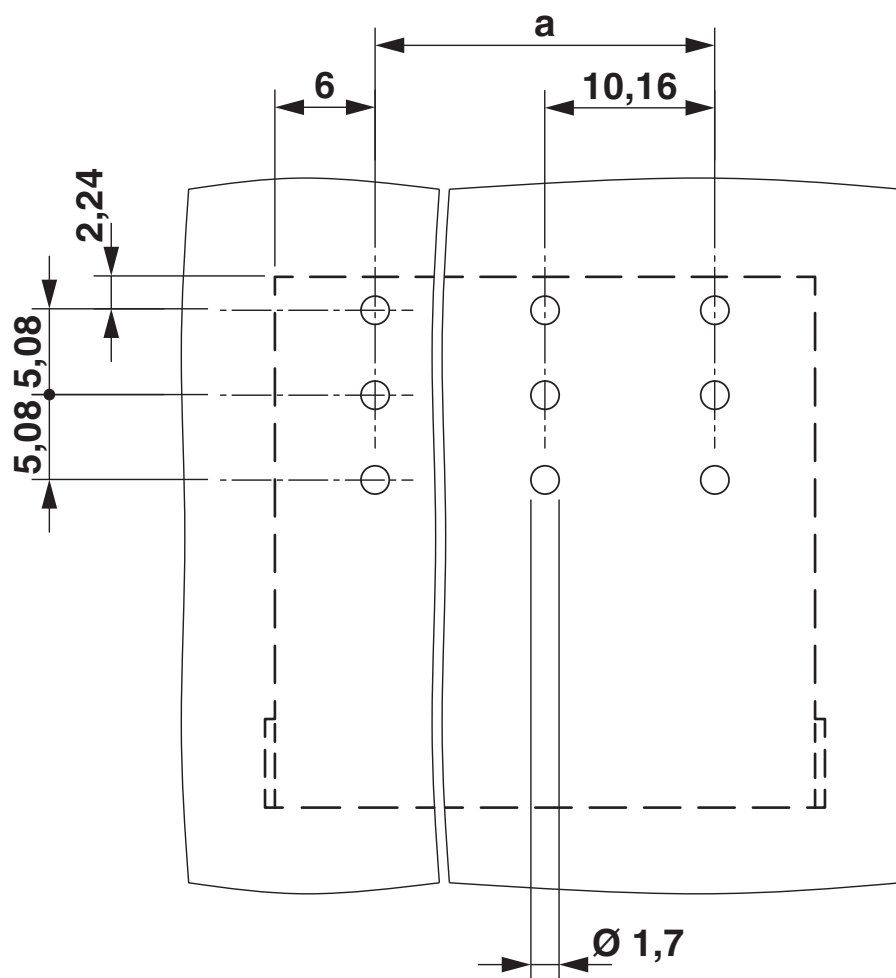
Bohrplan/Lötpadgeometrie
