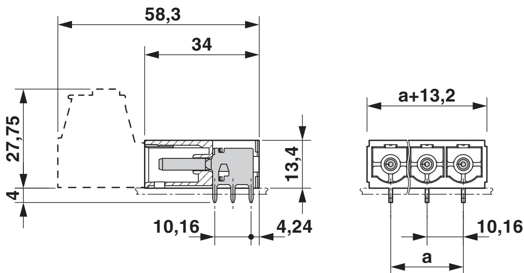
Maßzeichnung
