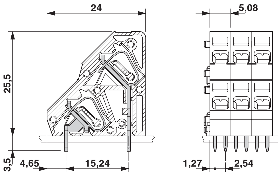
Maßzeichnung
