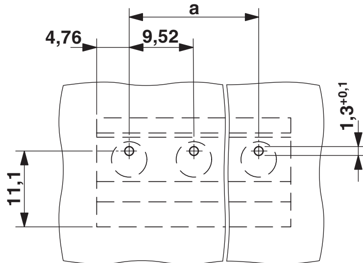
Bohrplan/Lötpadgeometrie
