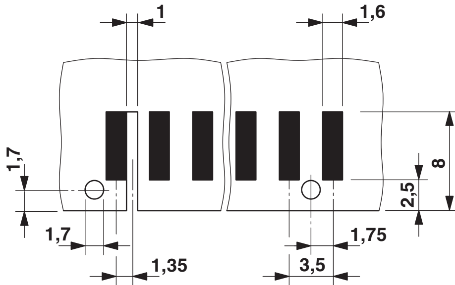
Bohrplan/Lötpadgeometrie
