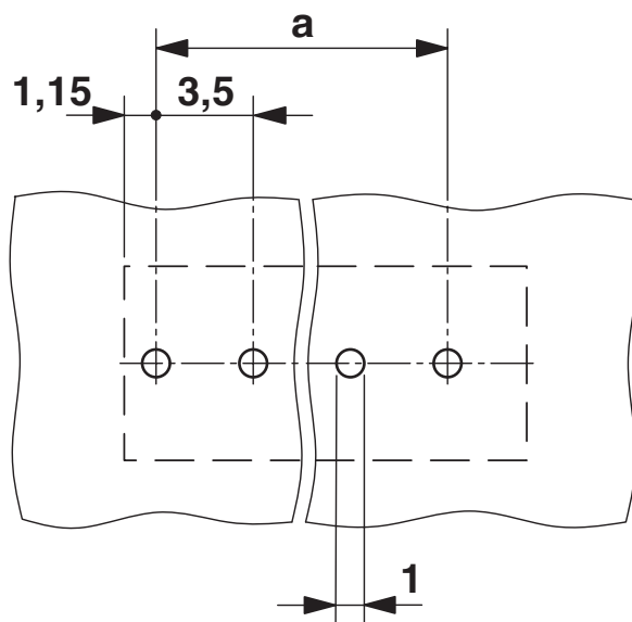
Bohrplan/Lötpadgeometrie
