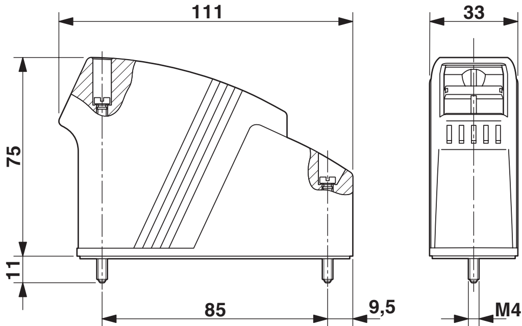
Maßzeichnung
