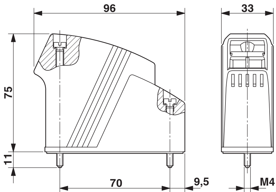
Maßzeichnung
