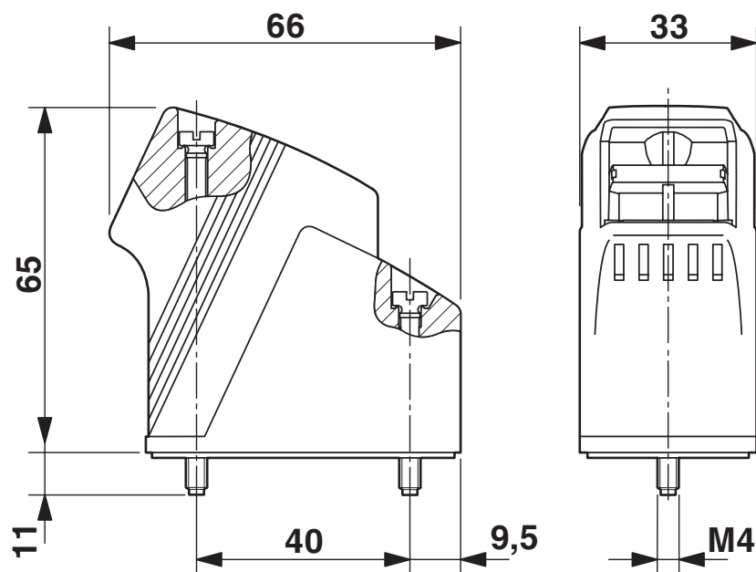
Maßzeichnung
