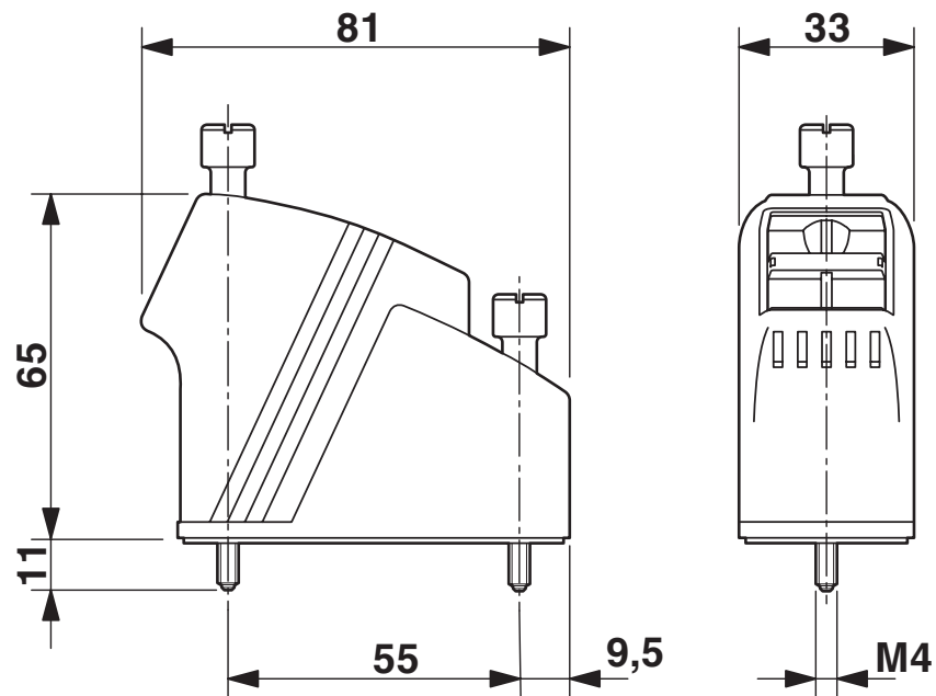
Maßzeichnung
