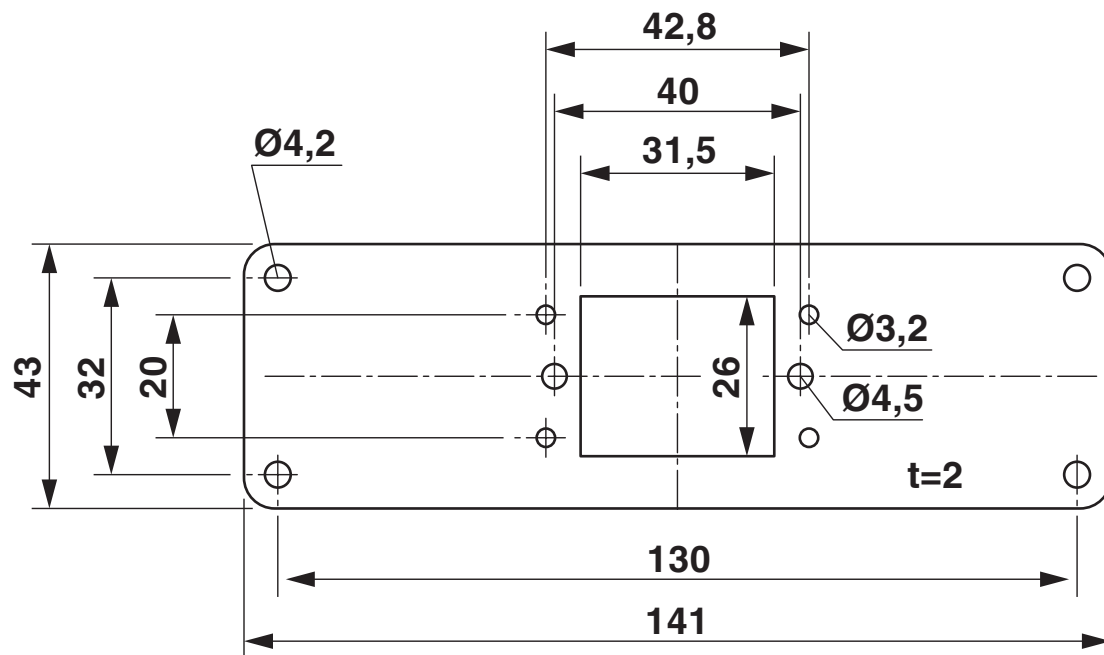
Maßzeichnung
