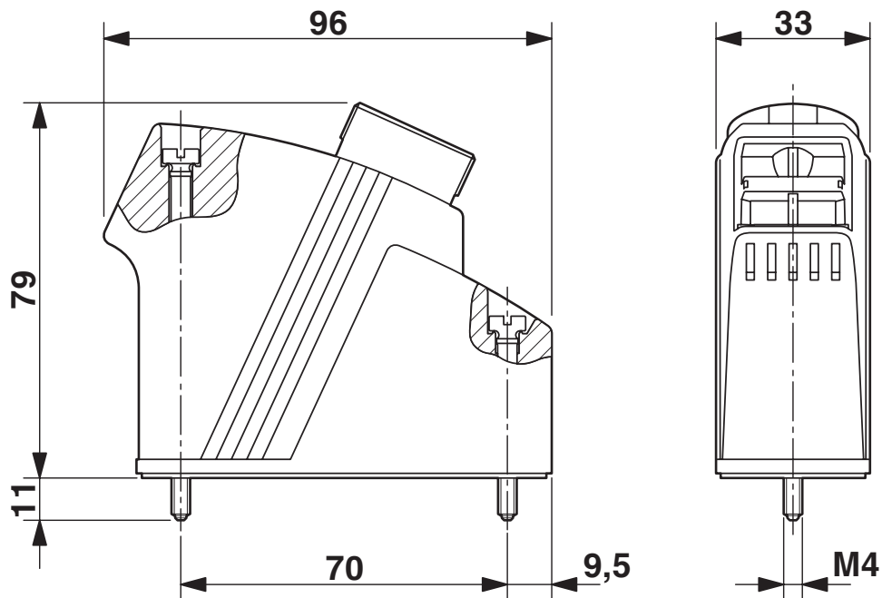
Maßzeichnung
