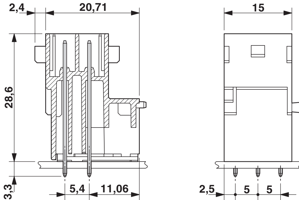
Maßzeichnung
