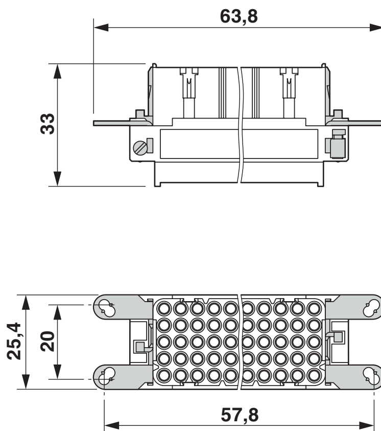
Maßzeichnung
