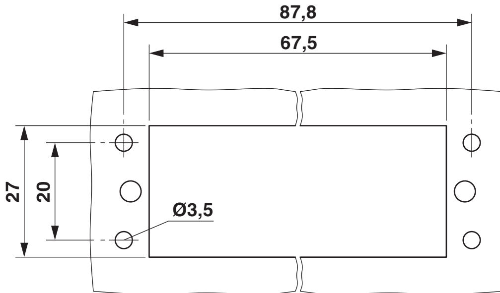
Maßzeichnung
