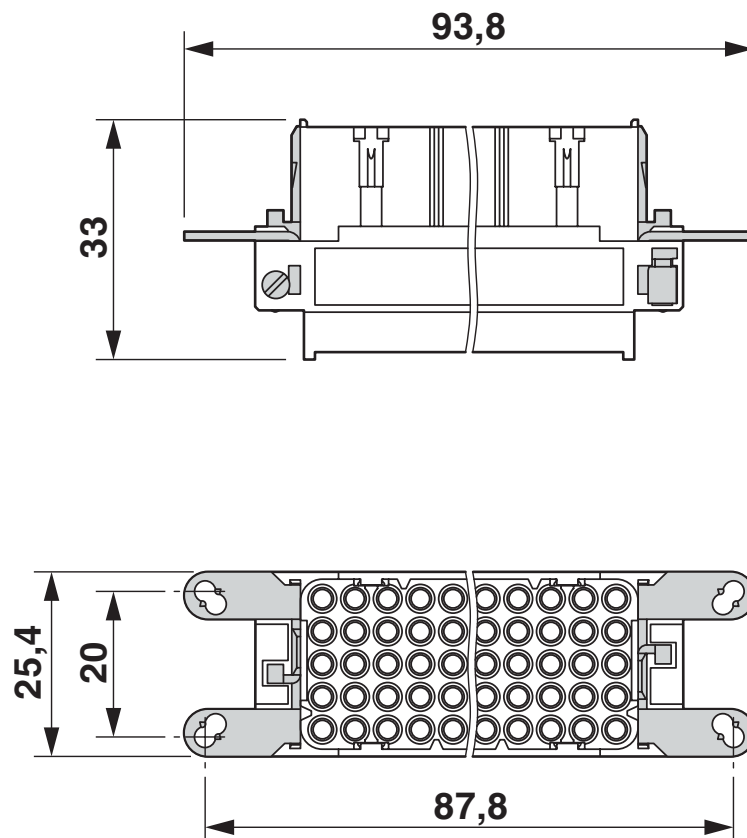
Maßzeichnung
