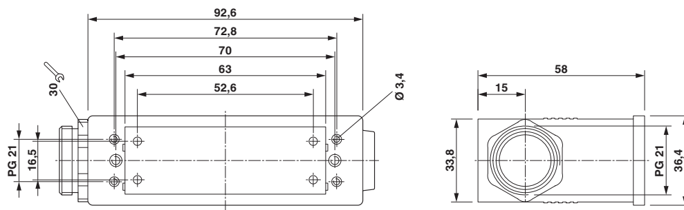
Maßzeichnung
