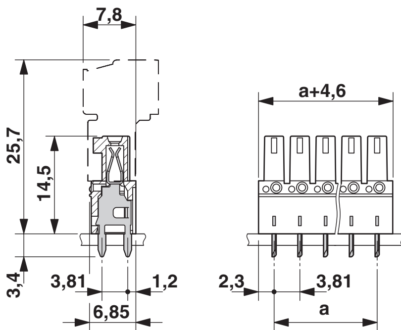
Maßzeichnung
