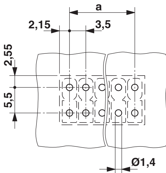
Bohrplan/Lötpadgeometrie
